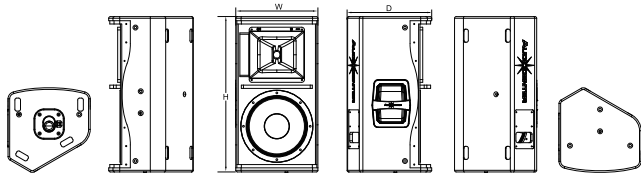
尺寸(W×H×D):300×568×309mm
